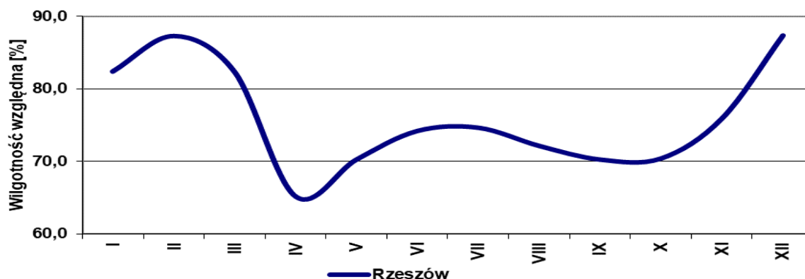
Rysunek 1-17 Przebieg średnich miesięcznych wartości wilgotności powietrza wyznaczonej przez model WRF/CALMET w strefie miasto Rzeszów w 2018 r.
