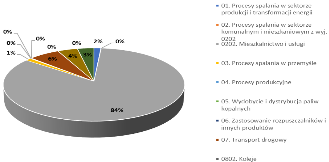
Rysunek 1-22 Udziały [%] poszczególnych rodzajów emisji z napływu na strefę miasto Rzeszów w łącznej emisji napływowej pyłu zawieszonego PM10
