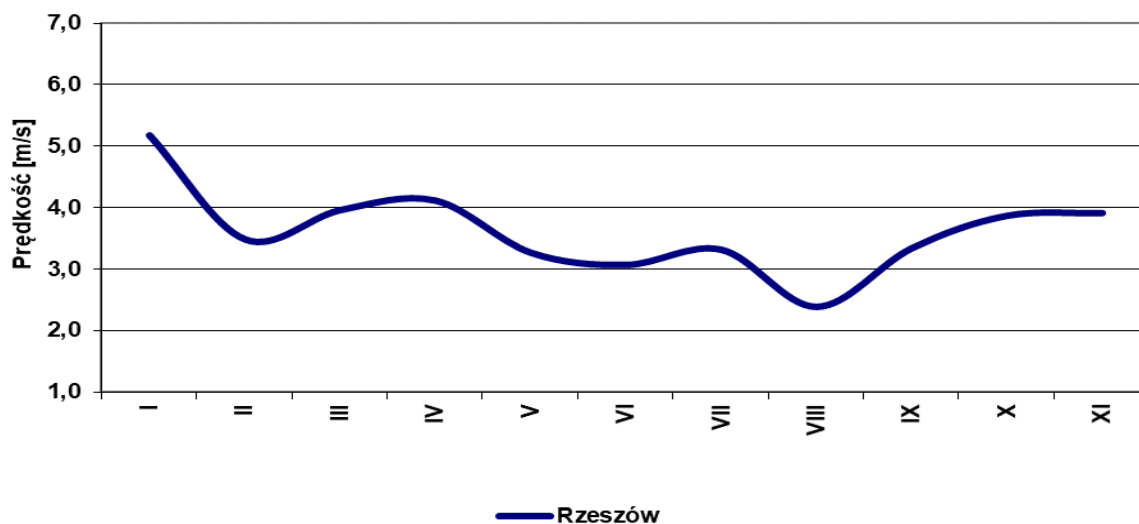
Rysunek 1-8 Średnia miesięczna prędkość wiatru wyznaczona przez model WRF/CALMET dla strefy miasto Rzeszów w 2018 r.
