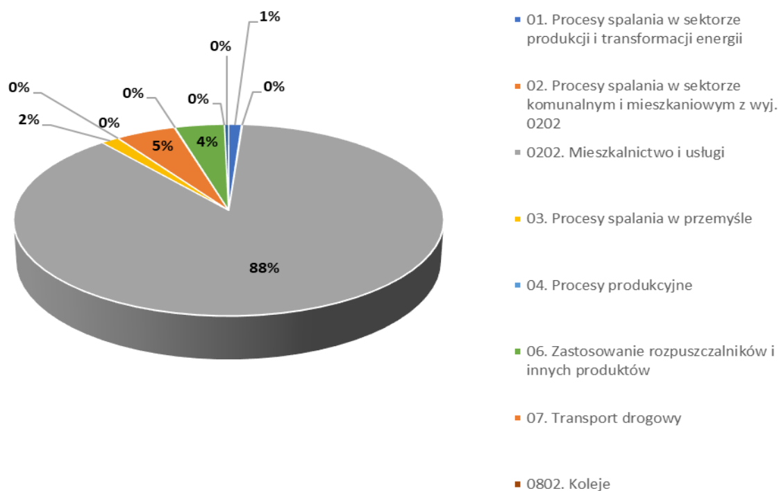
Rysunek 1-23 Udziały [%] poszczególnych rodzajów emisji z napływu na strefę miasto Rzeszów w łącznej emisji napływowej pyłu zawieszonego PM2,5
